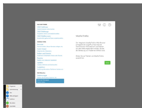
Hauptansicht - Startassistent
