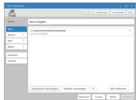
Datenquelle für Kopie auswählen
